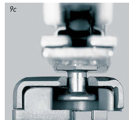
Illustration 9 : Systèmes de fermeture pour fenêtre (exemples) : Dispositif de verrouillage (9a), Tête champignon (9b), Renvoi d'angle (9c)
