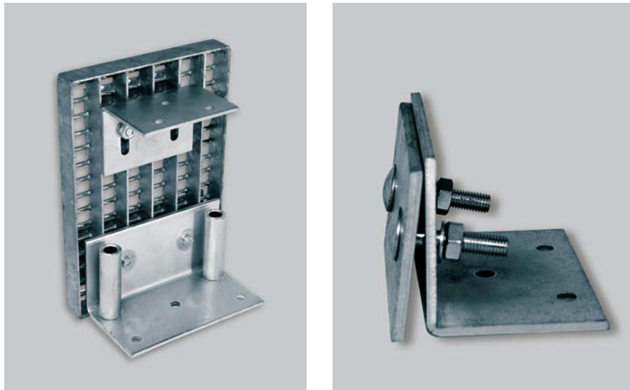
Illustration 16 : Exemples de dispositifs de fixation de grille
